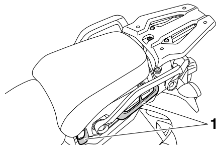
1. Spanngurt-Halterung
