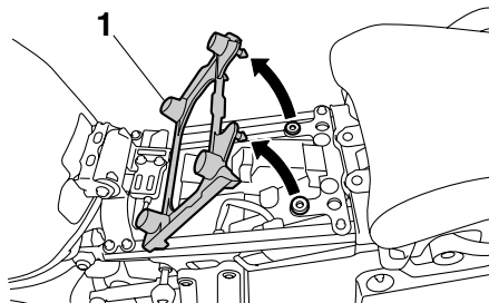
1. Fahrersitz-Höheneinsteller
